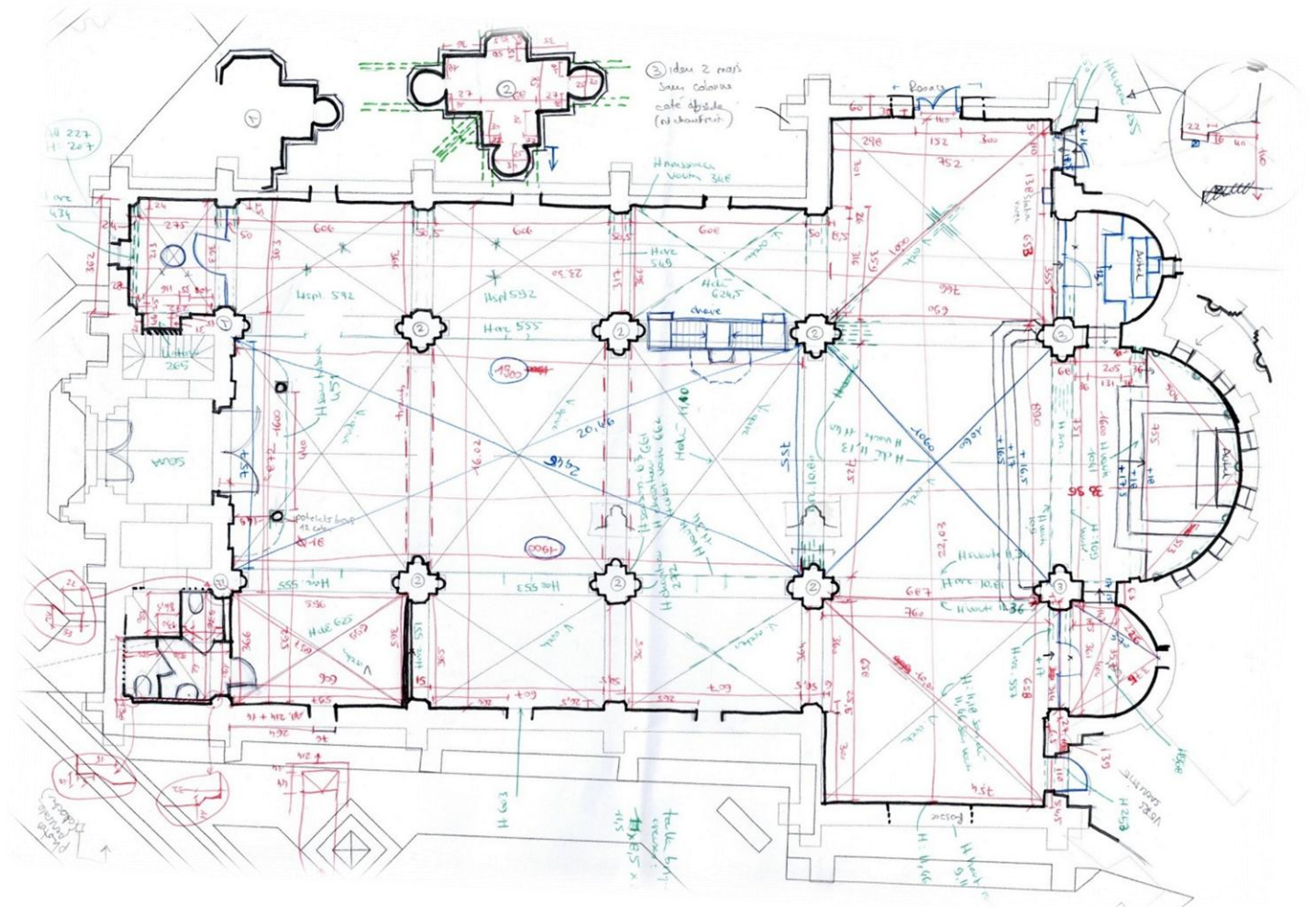
Relevé en plan de l'église
