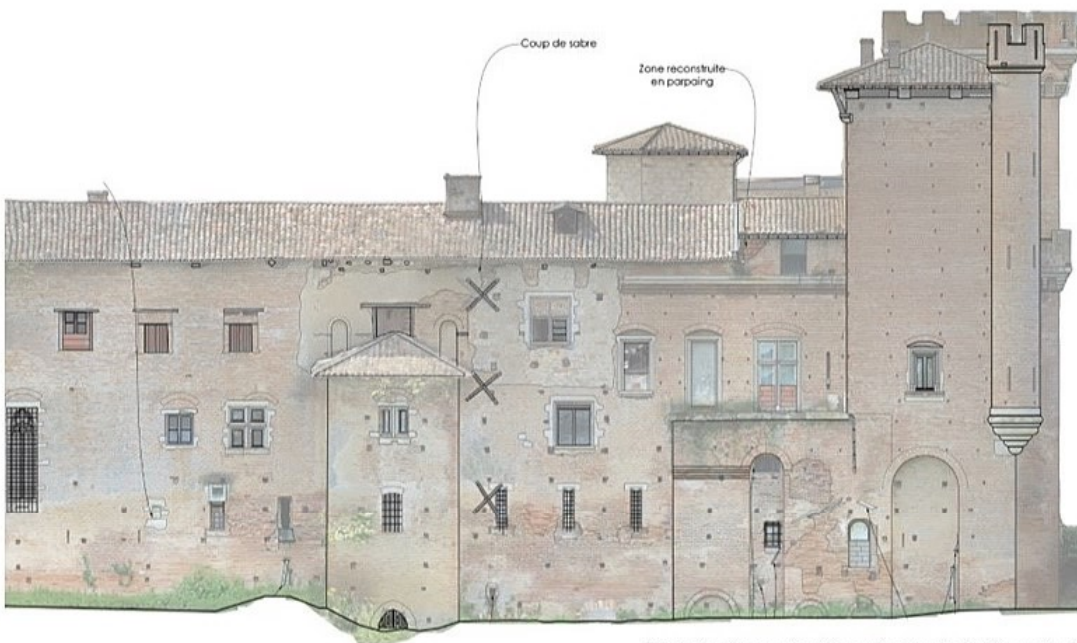
Etat des lieux et ortho-photo de la façade Est
