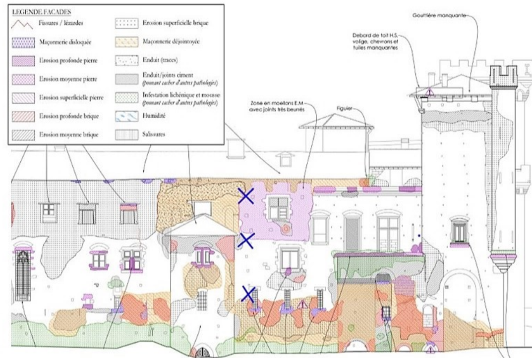
Cartographie des pathologies de la façade Est
