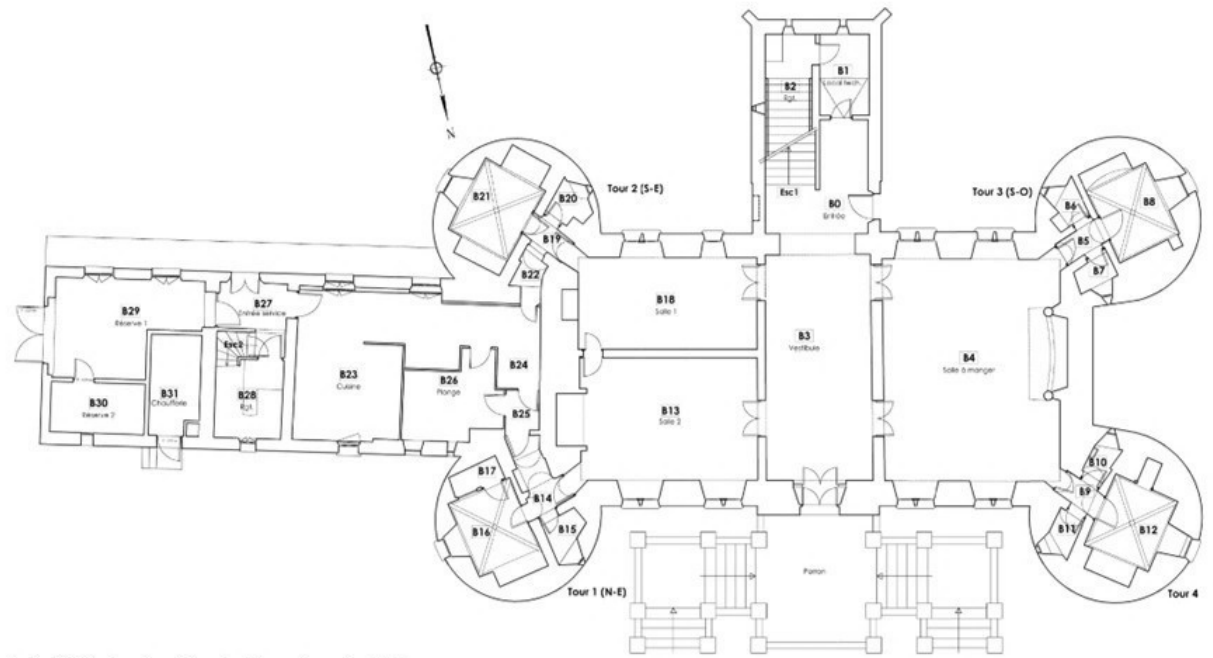
Relevé de l'état actuel (extrait) – plan du RDC
